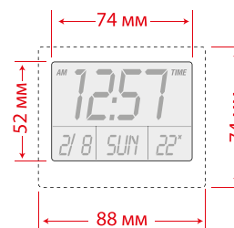
Габаритные размеры
