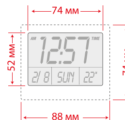
Габаритные размеры
